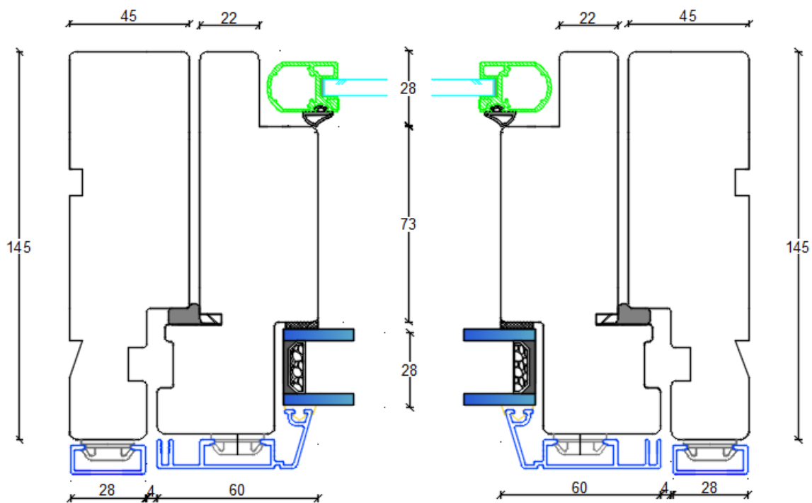
Vandret snit sidekarme/rammer:
