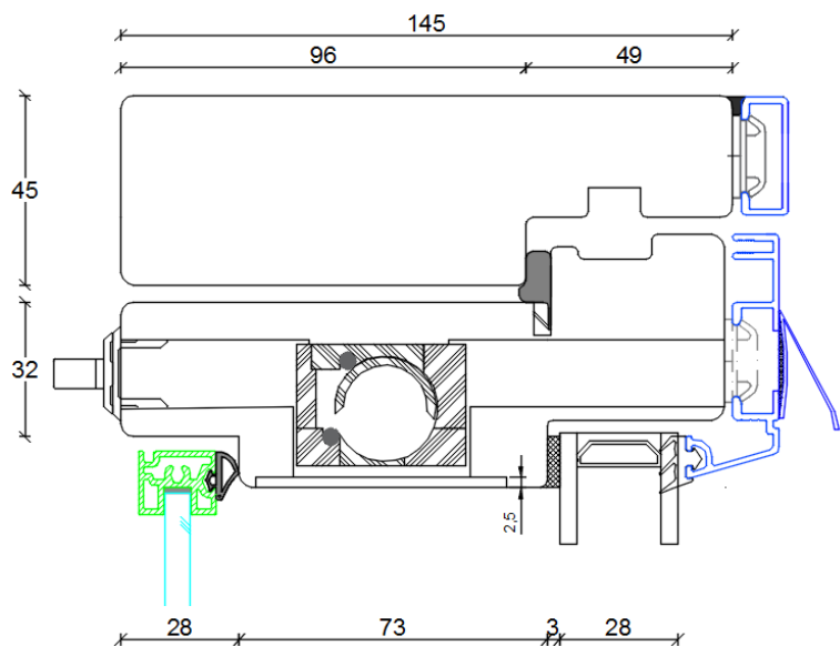
Lodret snit overkarm/ramme:
